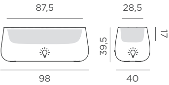
Dimensiones (cm)
