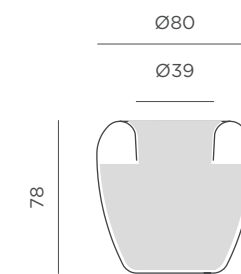
Dimensiones (cm)
