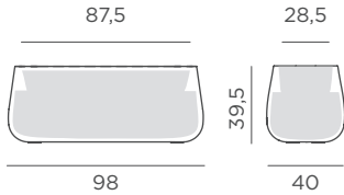
Dimensiones (cm)
