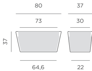
Dimensiones (cm)
