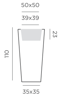
Dimensiones (cm)
