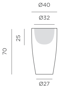
Dimensiones (cm)
