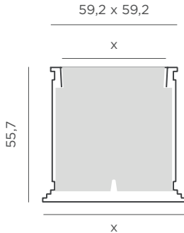
Dimensiones (cm)
