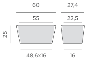
Dimensiones (cm)
