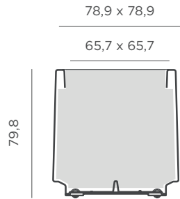
Dimensiones (cm)
