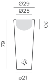
Dimensiones (cm)
