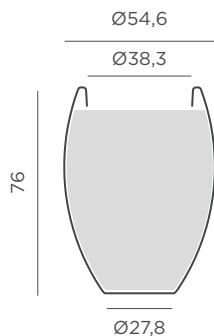
Dimensiones (cm)
