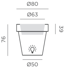
Dimensiones (cm)
