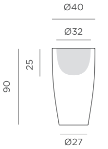
Dimensiones (cm)
