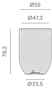
Dimensiones (cm)
