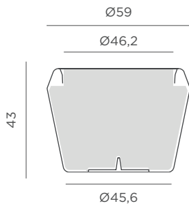
Dimensiones (cm)
