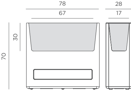
Dimensiones (cm)
