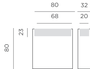
Dimensiones (cm)
