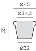
Dimensiones (cm)
