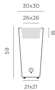
Dimensiones (cm)
