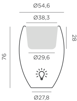
Dimensiones (cm)
