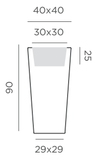
Dimensiones (cm)
