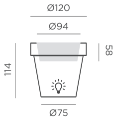
Dimensiones (cm)
